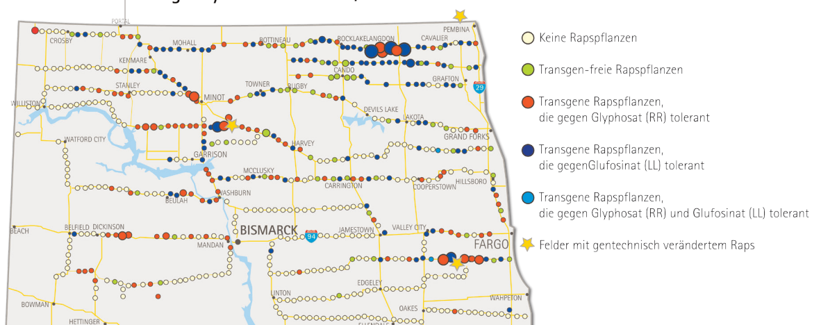
Abbildung 19: Ausbreitung von gentechnisch verändertem Raps entlang der Highways in North Dakota, US.
